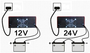
Figura 1: Exemplos de ligação em 12 Vdc e em 24 Vdc
