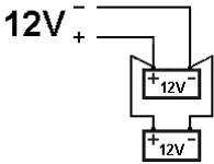
Figura 2: Ligação em paralelo
